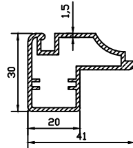
7034 0.624 kg/m
