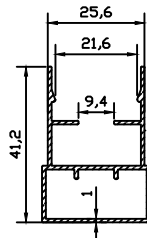
7043 0.428 kg/m
