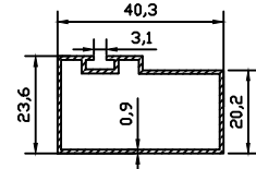
7045 0.331 kg/m
