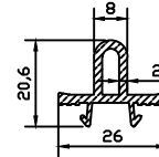
7012 0.345 kg/m
