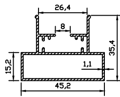
9524 0.563 kg/m
