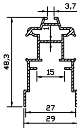
7042 0.480 kg/m
