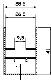
7044 0.425 kg/m
