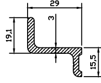
7006 0.500 kg/m
