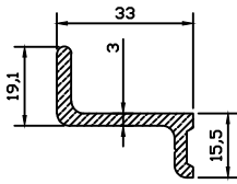
7005 0.532 kg/m
