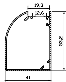
7046 0.568 kg/m
