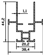
9525 0.509 kg/m
