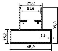
9523 0.552 kg/m
