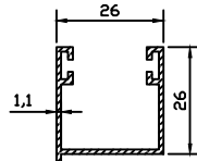
4001 0.291 kg/m
