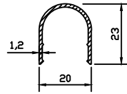
4004 0.181 kg/m
