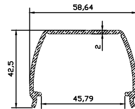
10122 0.867 kg/m
