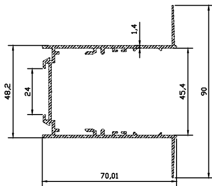
10230 1.027 kg/m
