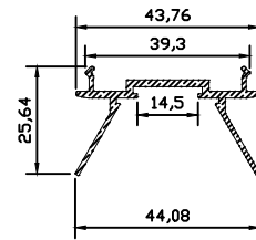
10066 0.377 kg/m
