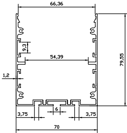
10346 1.306 kg/m
