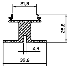
10235 0.791 kg/m
