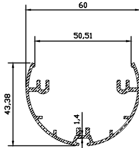
10263 0.743 kg/m
