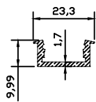
10169 0.192 kg/m
