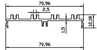
10342 0.688 kg/m
