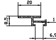
6077 0.160 kg/m
