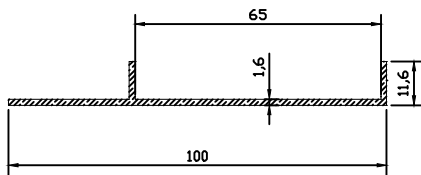
10479 0.519 kg/m
