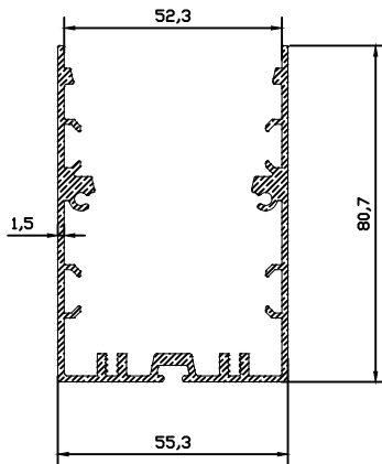
10068 1.447 kg/m
