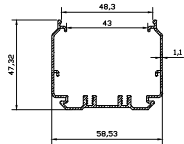
10351 0.653 kg/m
