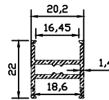
10429 0.306 kg/m
