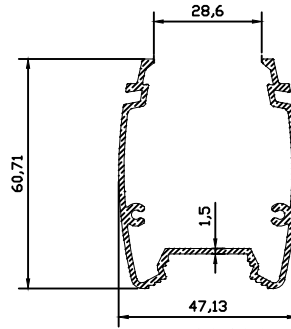
10122 0.867 kg/m
