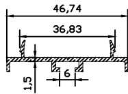
10195 0.295 kg/m
