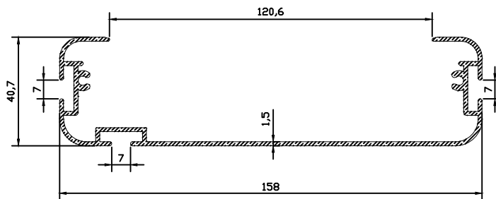
10196 1.401 kg/m
