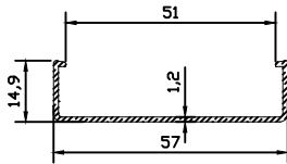
10467 0.282 kg/m
