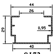
9172 0.323 kg/m
