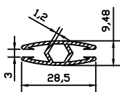
9220 0.254 kg/m
