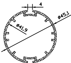
10388 0.743 kg/m
