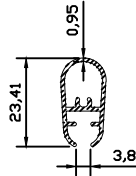
9798 0.189 kg/m
