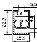
9535 0.298 kg/m
