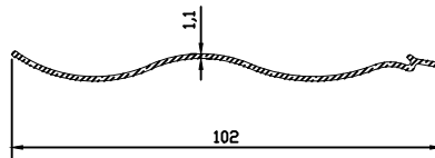
9781 0.322 kg/m
