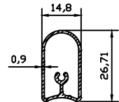
9560 0.224 kg/m
