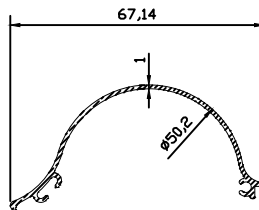
10040 0.276 kg/m
