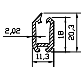
9096 0.242 kg/m
