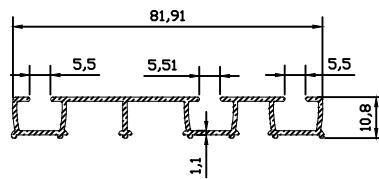
10354 0.515 kg/m
