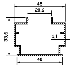
9085 0.422 kg/m
