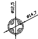
9800 0.262 kg/m
