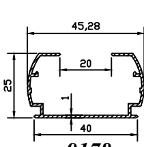
9178 0.325 kg/m
