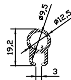
9794 0.227 kg/m
