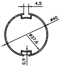
10454 0.439 kg/m
