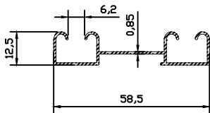
9772 0.287 kg/m
