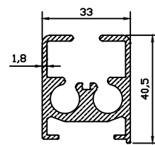
9333 1.150 kg/m
