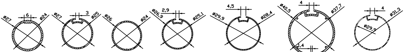
9115 0.339 kg/m
