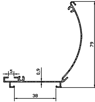
10455 0.504 kg/m
