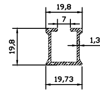
10353 0.266 kg/m
