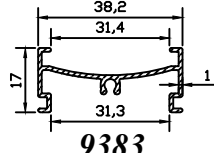
9383 0.256 kg/m
