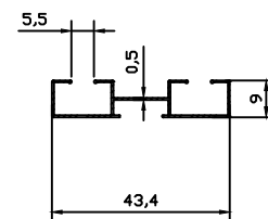
5166 0.133 kg/m
