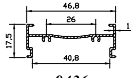
9436 0.279 kg/m
