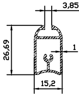
9775 0.281 kg/m
