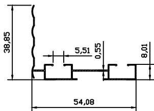
5168 0.187 kg/m
