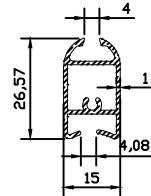
9813 0.273 kg/m
