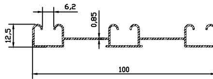
9773 0.461 kg/m
