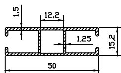
9537 0.517 kg/m
