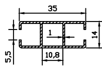
9054 0.287 kg/m
