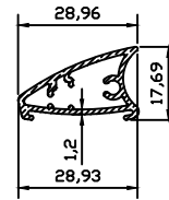
10456 0.328 kg/m
